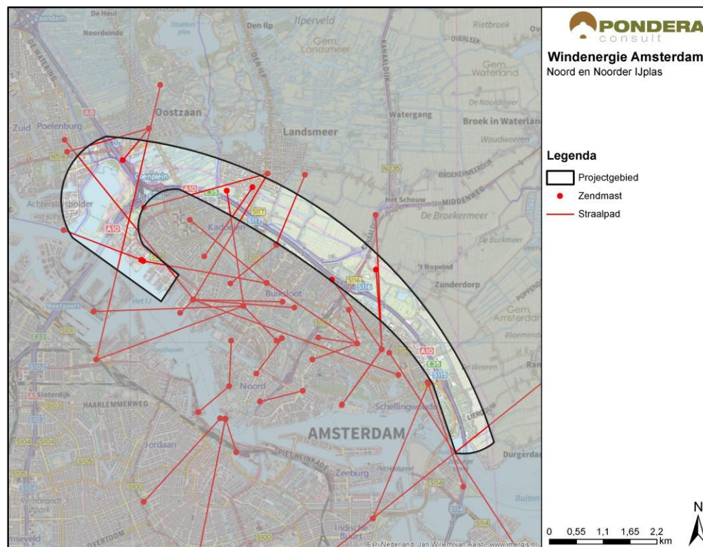
Figuur 2.18 Straalpaden
